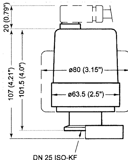
Rys. 1. Schemat z wymiarami - głowica próżniowa typu Full Range DN 25 ISO-KF, 1000-5x10e-9 mbar.
